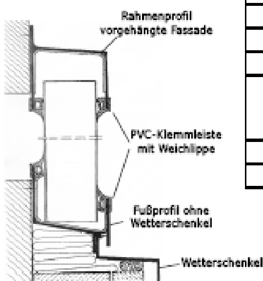
für vorgehängte Fassade
