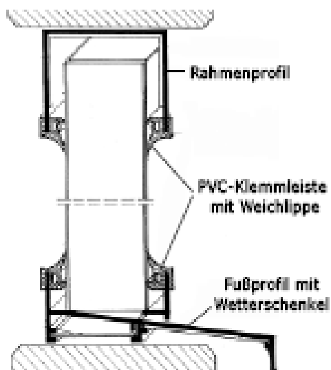
für Wandverglasung in Laibung
